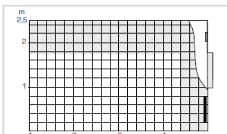
Buitentemperatuur: ±0°C, binnentemperatuur +20°C Luchtdoorlaat: 10 ltr/sec, radiatorcapaciteit 400W
