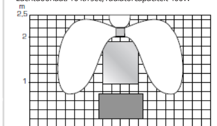
Buitentemperatuur: -20°C, binnentemperatuur +20°C Luchtdoorlaat: 10 ltr/sec, radiatorcapaciteit 400W
