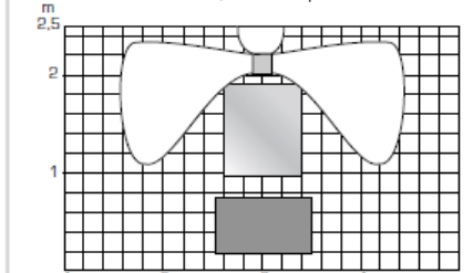
Buitentemperatuur: ±0°C, binnentemperatuur +20°C Luchtdoorlaat: 10 ltr/sec, radiatorcapaciteit 400W
